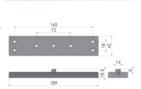
RF Puerta cortafuego / Fireproof door 1820 RF
